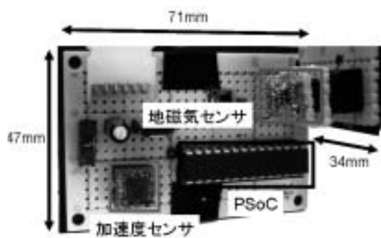
インテリジェント歩数計の外観と構成
