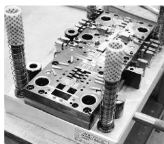
高度な穴加工が施されたプレート。この金型に帯状の金属を通すと、右写真のようなコネクタが連続した端子部品ができる
